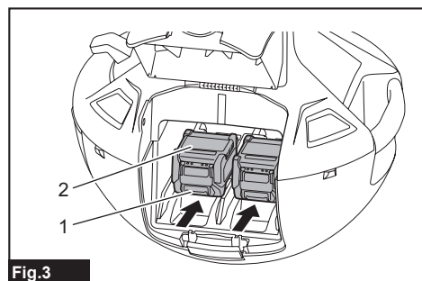
Fig.3 ► 1. Bouton 2. Batterie
