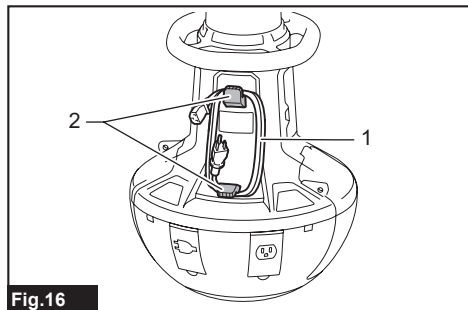
► 1. Cordon d'alimentation 2. Crochet pour cordon d'alimentation
