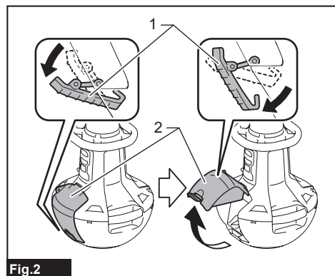
Fig.2 ► 1. Verrou du couvercle 2. Couvercle de batterie
